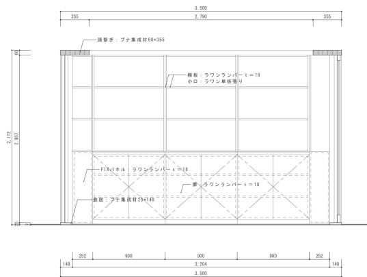
F-51B A断面図 S=1:20
