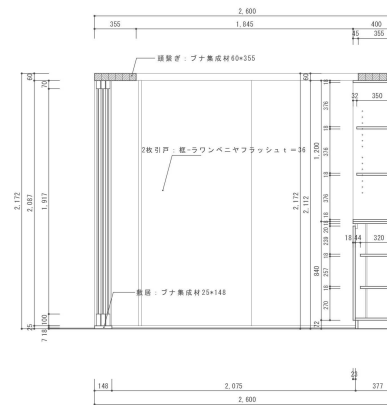
F-51B B断面図 S=1:20
