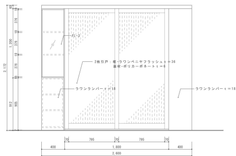
F-51B a変図 S=1:20
