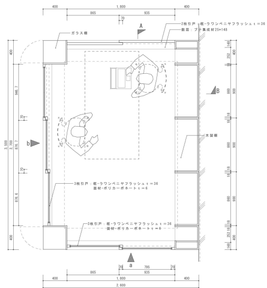
F-51B 平面図 S=1:20
