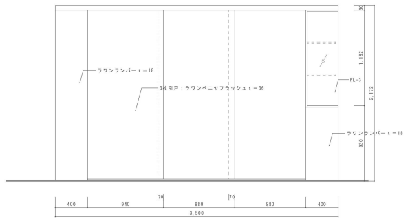
F-51A a断面図 S=1:20
