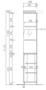
F-51A C断面図 S=1:20
