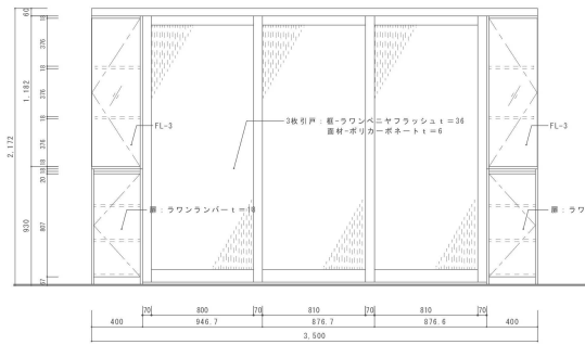
F-51A b断面図 S=1:20
