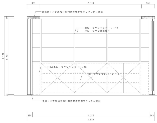
F-51A A断面図 S=1:20
