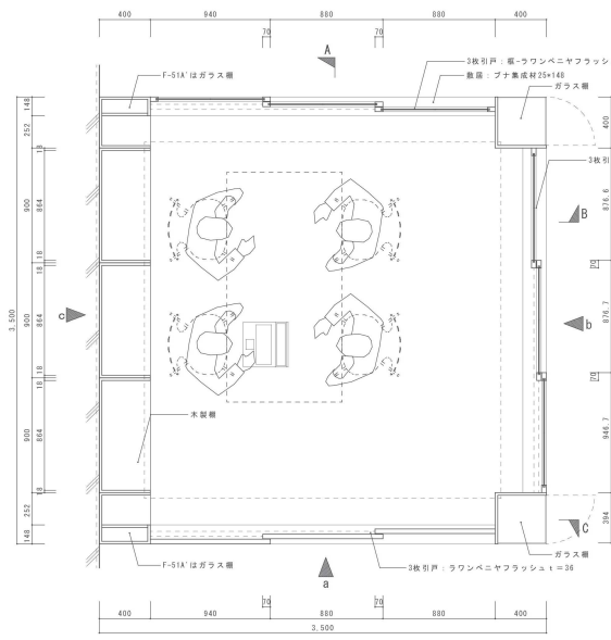
F-51A 平面図 S=1:20
