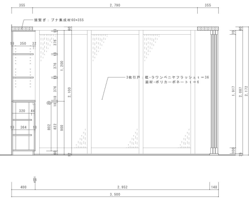
F-51A B断面図 S=1:20
