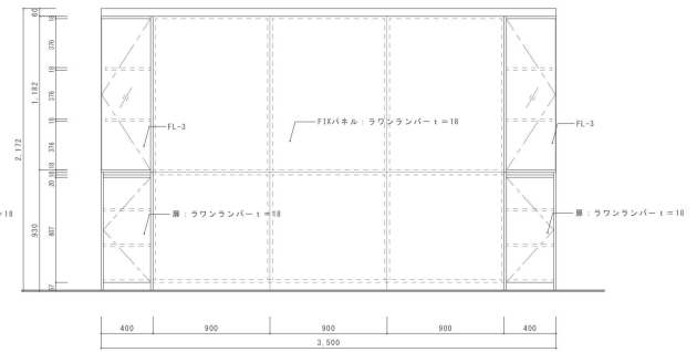
F-51A' b断面図 S=1:20
