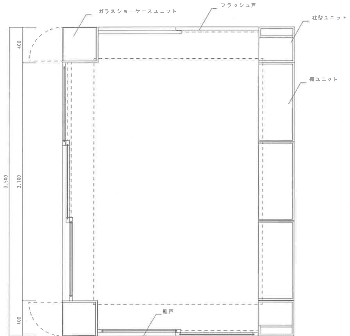
Bタイプ (壁付配置) 平面図 S=1:20
